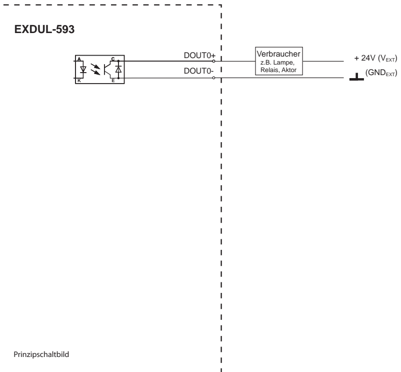
Gratik 18.2 Beschaltung des Optokoppler-Ausgangs
