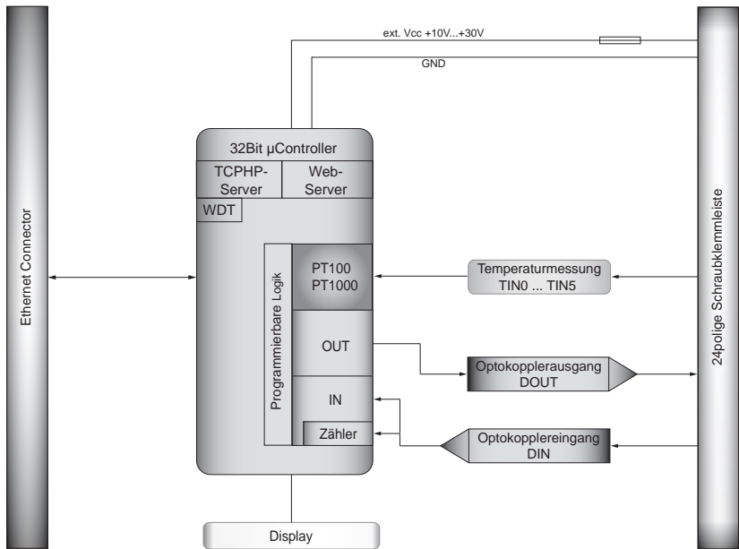
Grafik 3.1 Blockschahtbild EXDUL-593E
