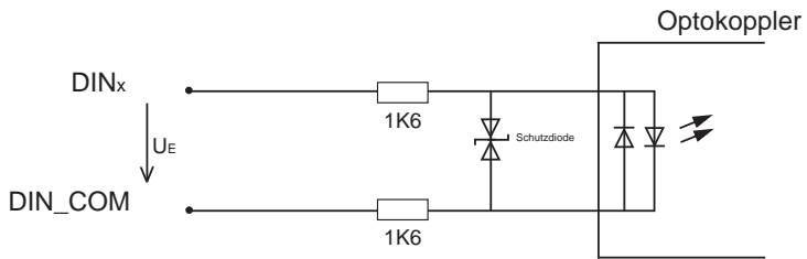
Abb. 7.2 Eingangsbeschaltung
