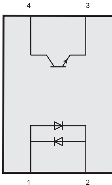
Abb. 7.1 Pinning Eingangsoptokoppler
