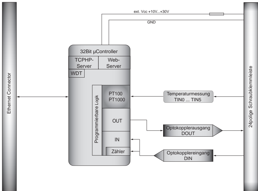
Grafik 3.2 Blockschahtbild EXDUL-593S
